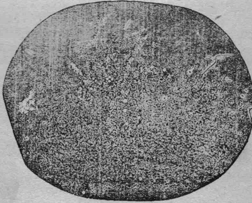
Bildo 1ª.—Nebulozo.
