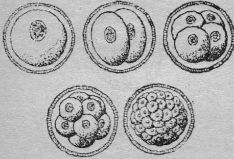
Bildo 18 a
