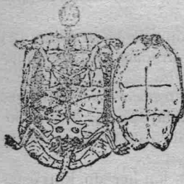
Bildo 5 a .
