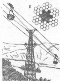
D.—Detalo. Aerakablo.
