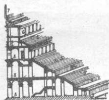
Sekcio vertikala, laŭ la plej granda akso, de la Anfiteatro Flavia. Romo.
