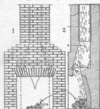
Faco k. sekcio de kameno.
