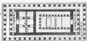
Plano de greka templo kun interna k. ekstera peristilo.
