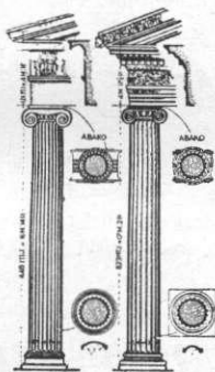
Greka k. romana jonika ordo.
