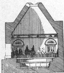
Sekcio de frigidario en pompeja domo.
