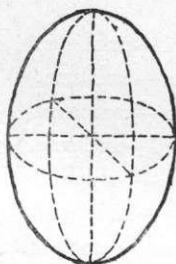
Elipso k. elipsoido.
