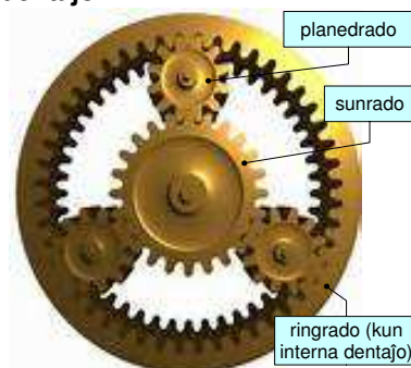
dentrada planedaro
