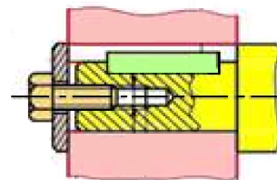
stifta kuplilo
