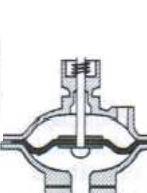
membrana pumpilo
