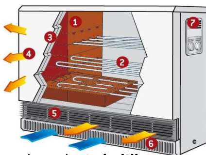
akumulanta hejtilo proviza nur dum noktotaŝarifaĵoj (interne brikoj akumulas varmo danke al termika inercio)
