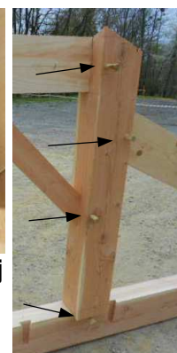
ĉarpentaj kejloj
