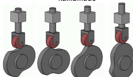
vertikalan movon okazigi per rotacio de kamo
