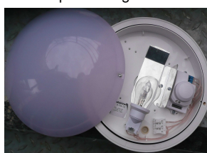
movdetektila lampo per altfrekvenca (lampo de la kastelo Greziljono)
