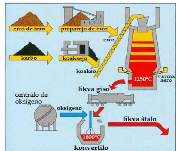
altforno en gisejo
