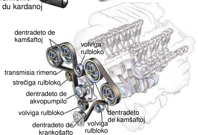
perrimena transmisiilo (motoro V6 24 valvoj)
