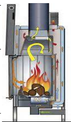
brulkamero en kamenstovo
