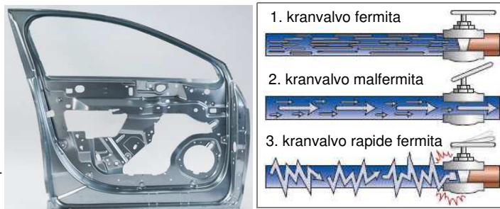
premfrapo kaŭze de kranvalvo
