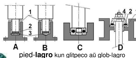
ped-lagro kun glitpeco aŭ glob-lagro
