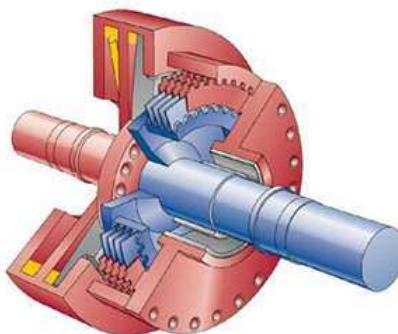
multdiska hidraŭlika kluĉilo
