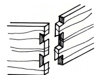
hirundvosta junto
