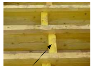
stego inter solivoj
