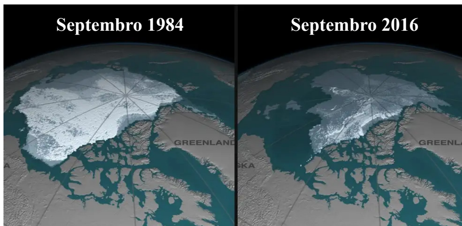
Grafika komparo de la fandiĝo de la Norda Poluso dum la lastaj jardekoj.
